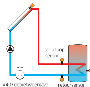
V40/debietweergave retoursensor
